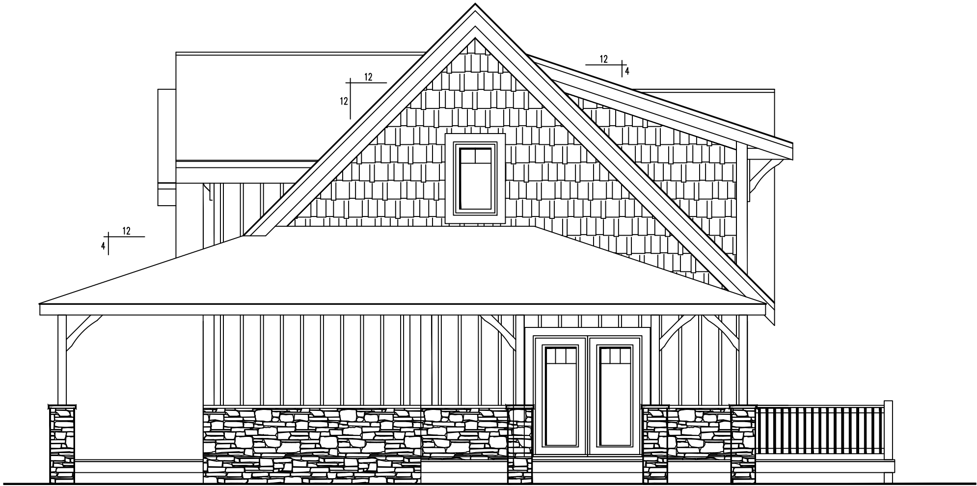
RIGHT ELEVATION
