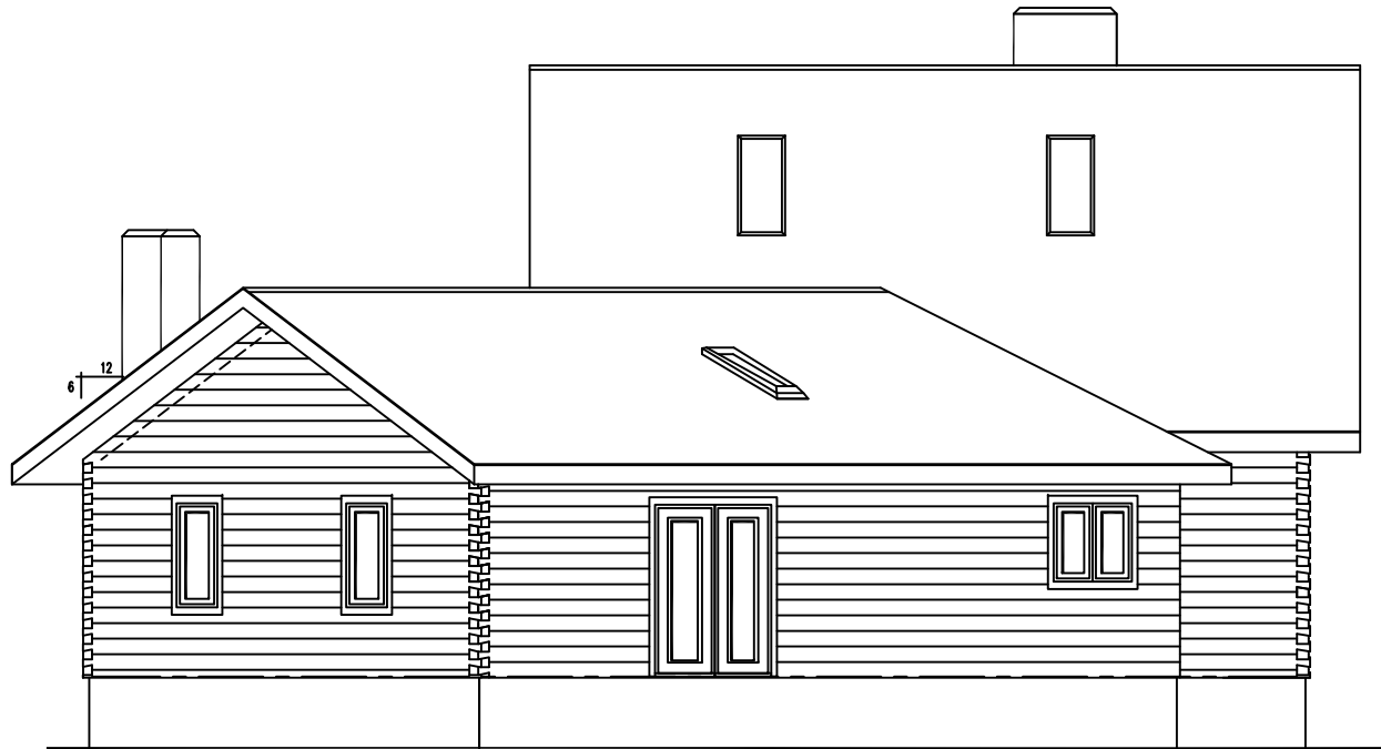
RIGHT ELEVATION
