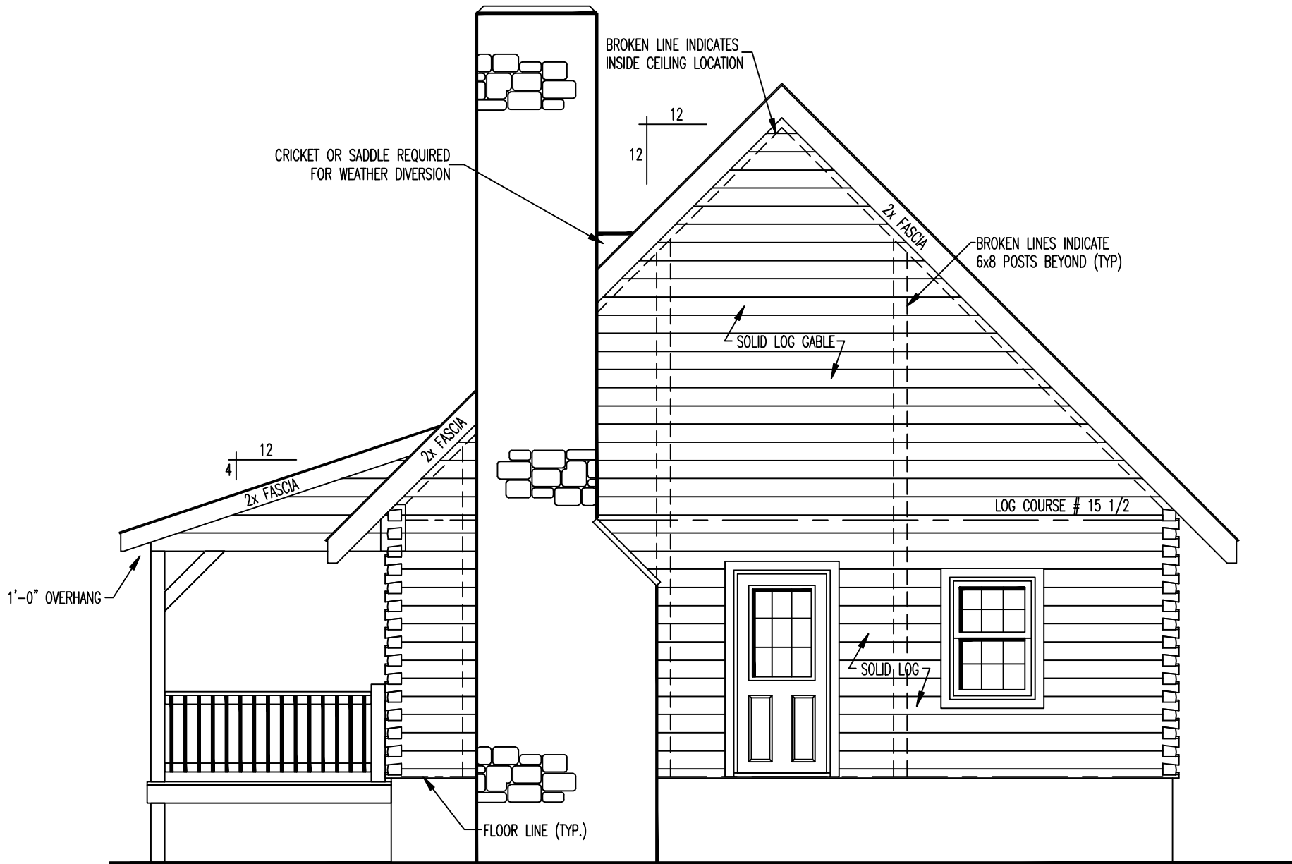
RIGHT ELEVATION
