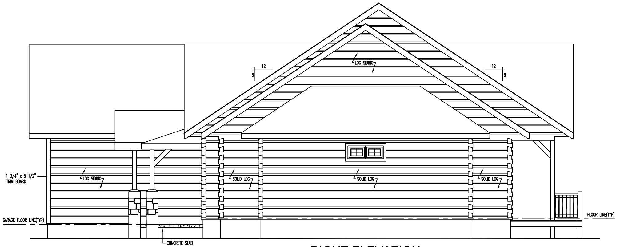
RIGHT ELEVATION
