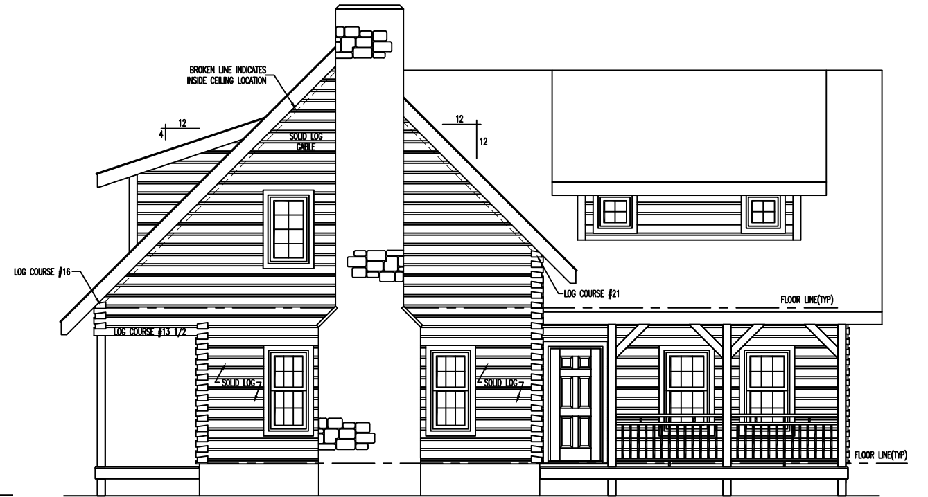
RIGHT ELEVATION
