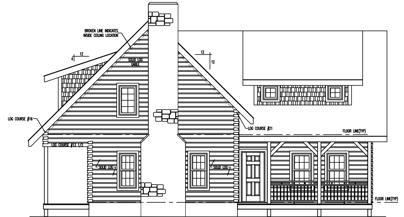
RIGHT ELEVATION
