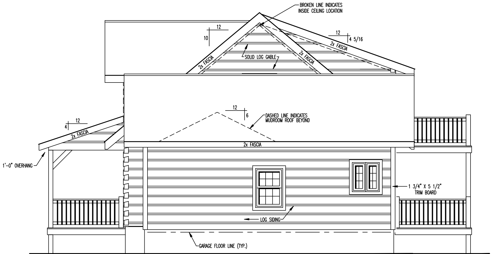
RIGHT ELEVATION
