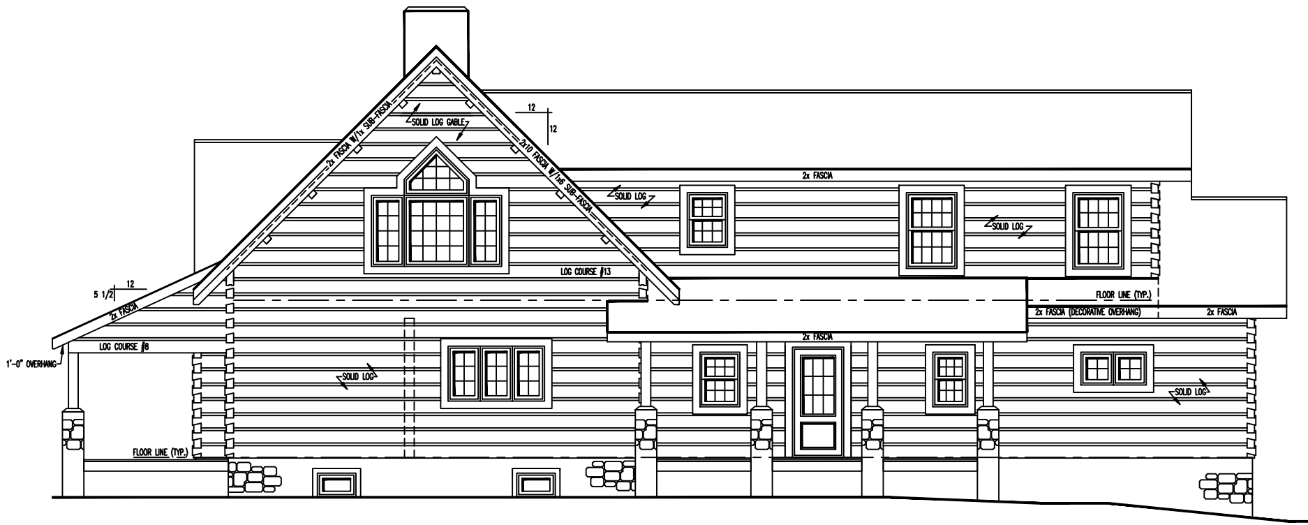
RIGHT ELEVATION
