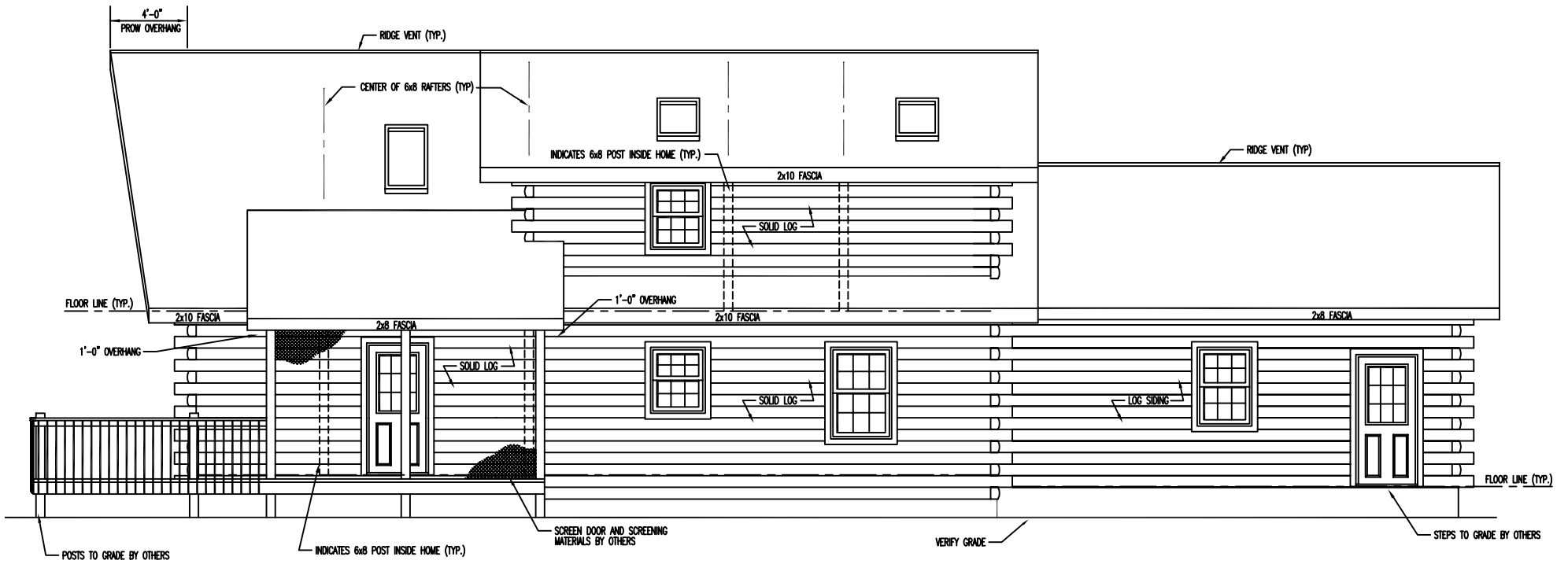
RIGHT ELEVATION
