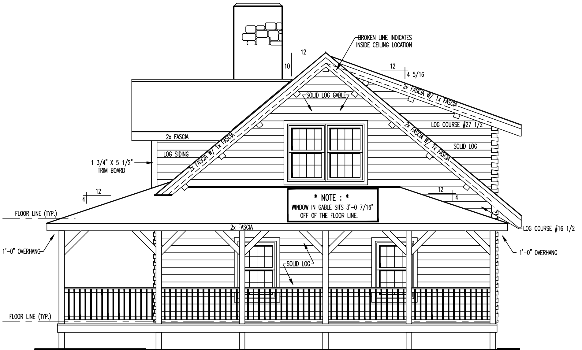
RIGHT ELEVATION
