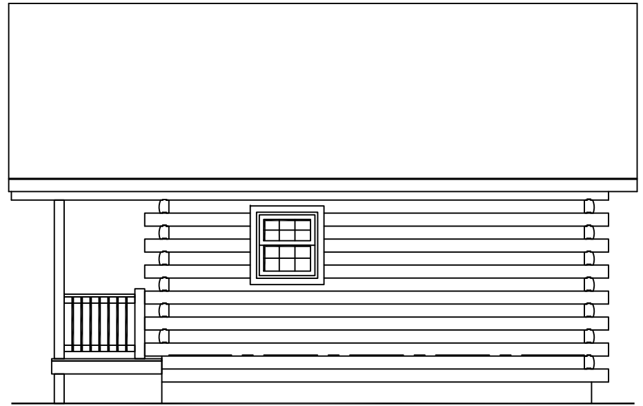
RIGHT ELEVATION
