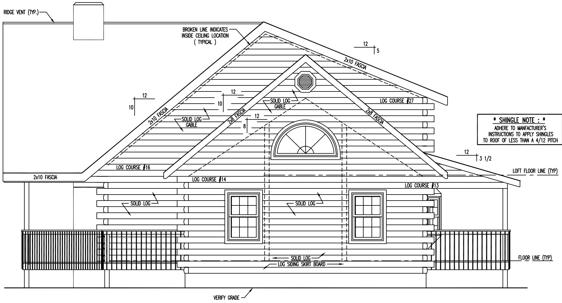
RIGHT ELEVATION
