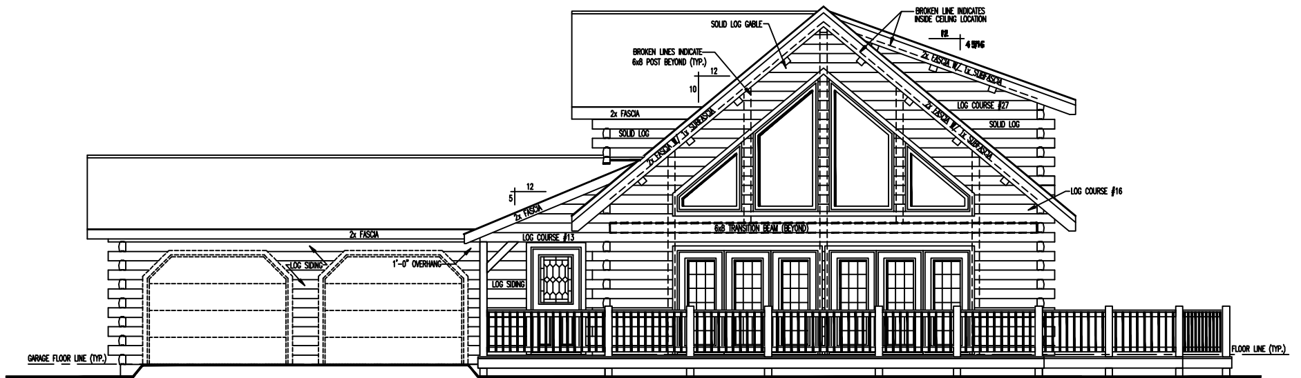
RIGHT ELEVATION
