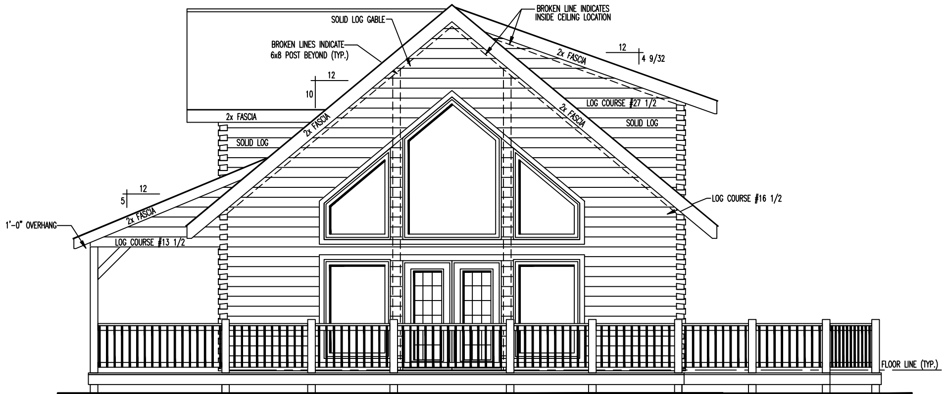
RIGHT ELEVATION
