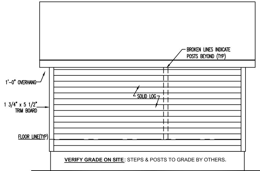
RIGHT ELEVATION
