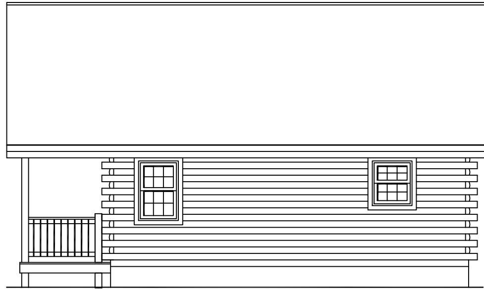
RIGHT ELEVATION
