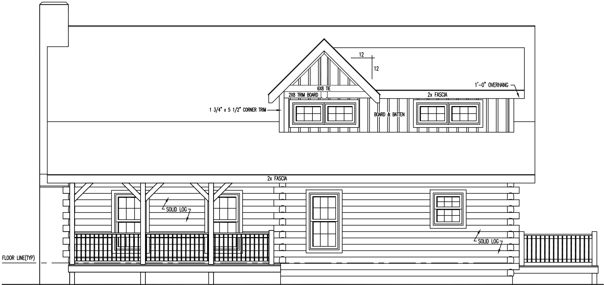
RIGHT ELEVATION
