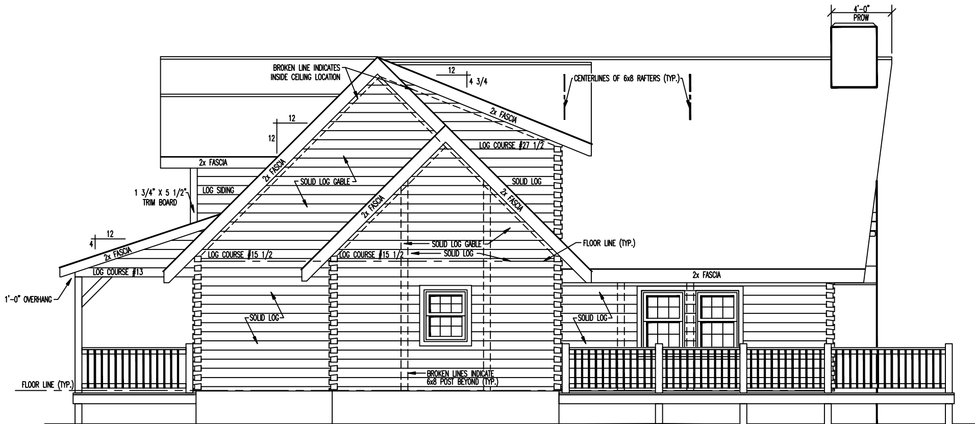
RIGHT ELEVATION
