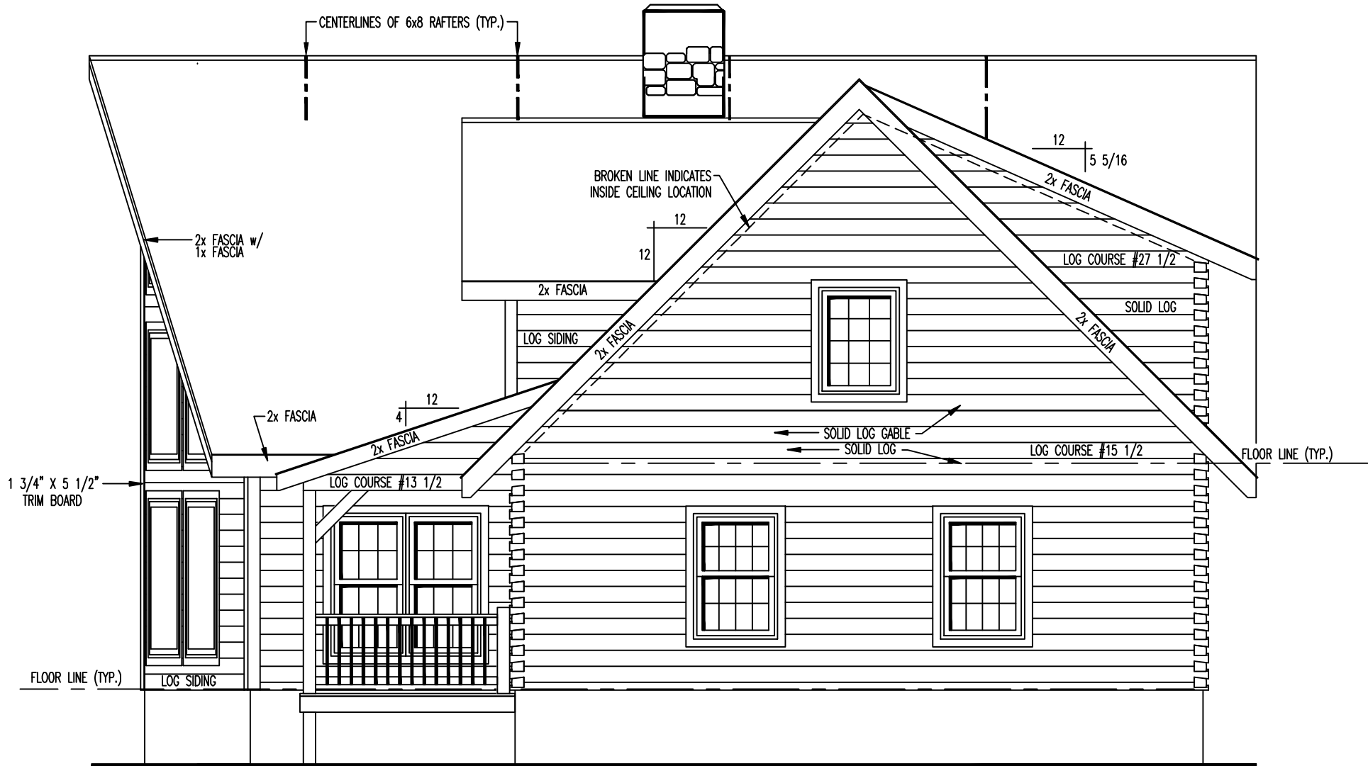
RIGHT ELEVATION
