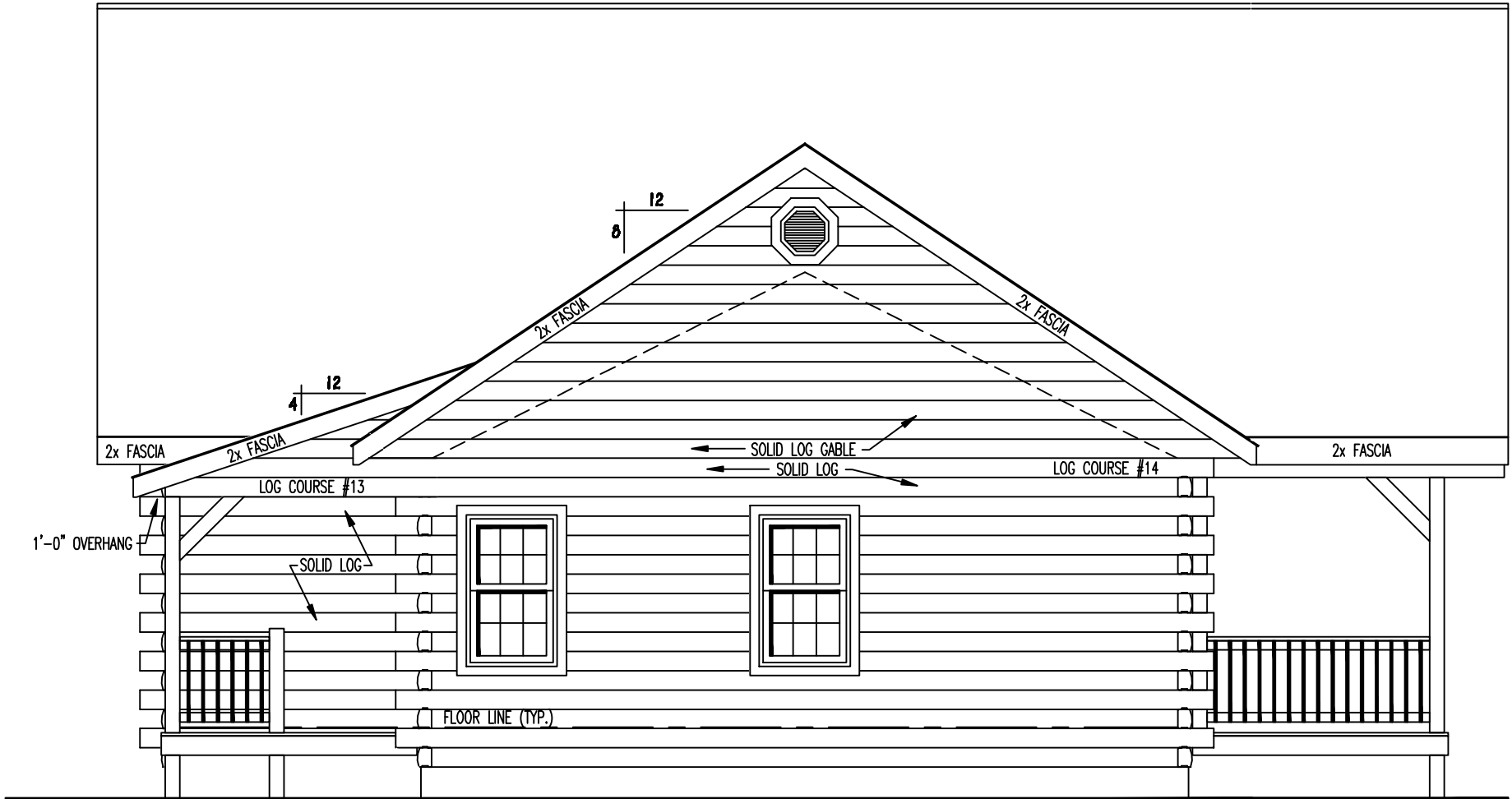
RIGHT ELEVATION
