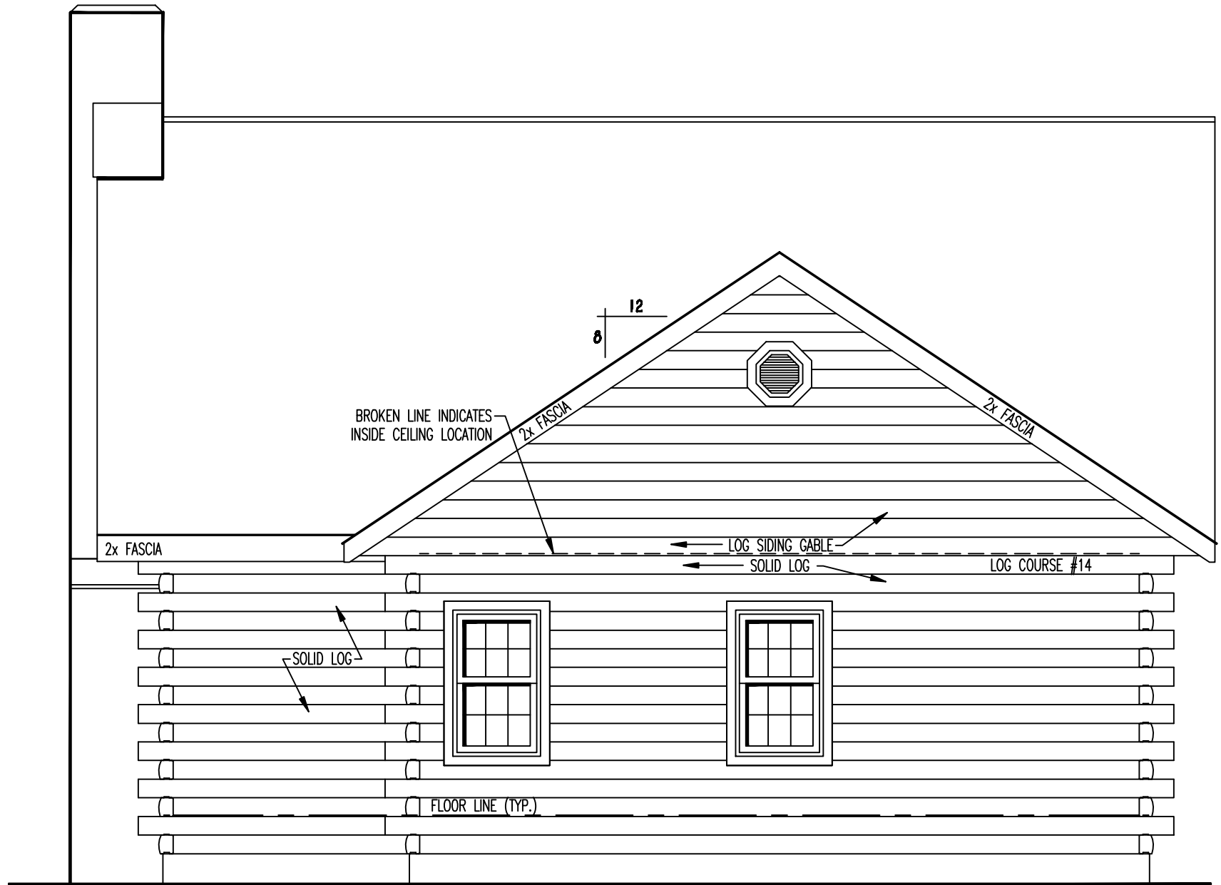
RIGHT ELEVATION
