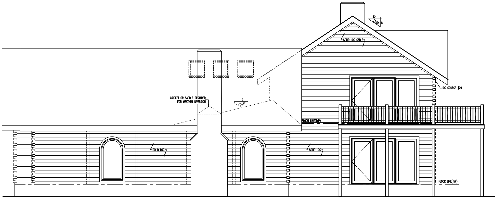
RIGHT ELEVATION
