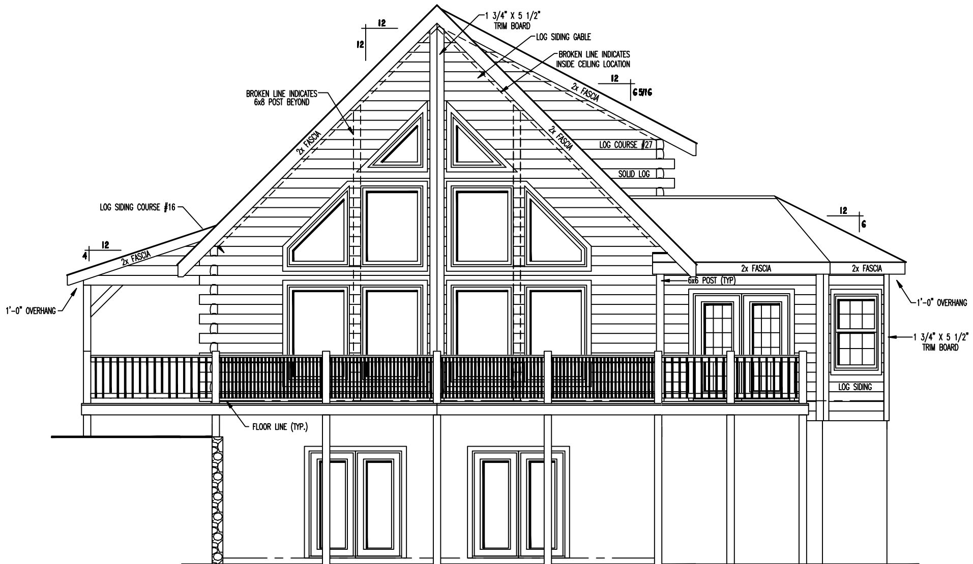
RIGHT ELEVATION
