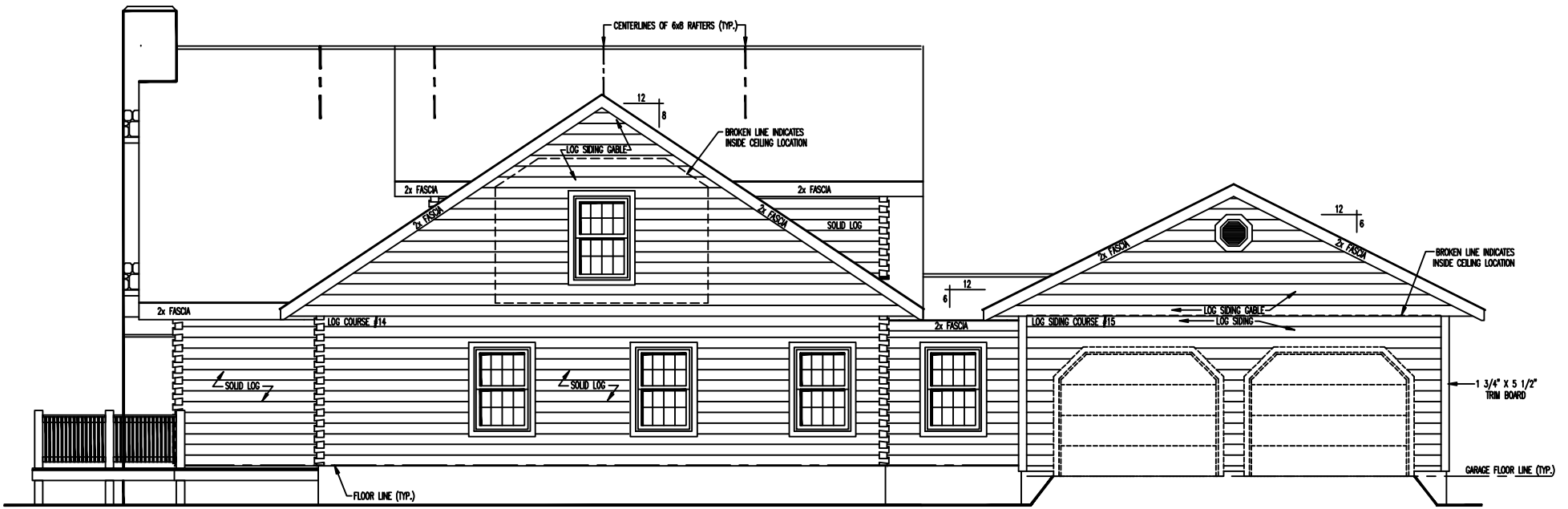
RIGHT ELEVATION
