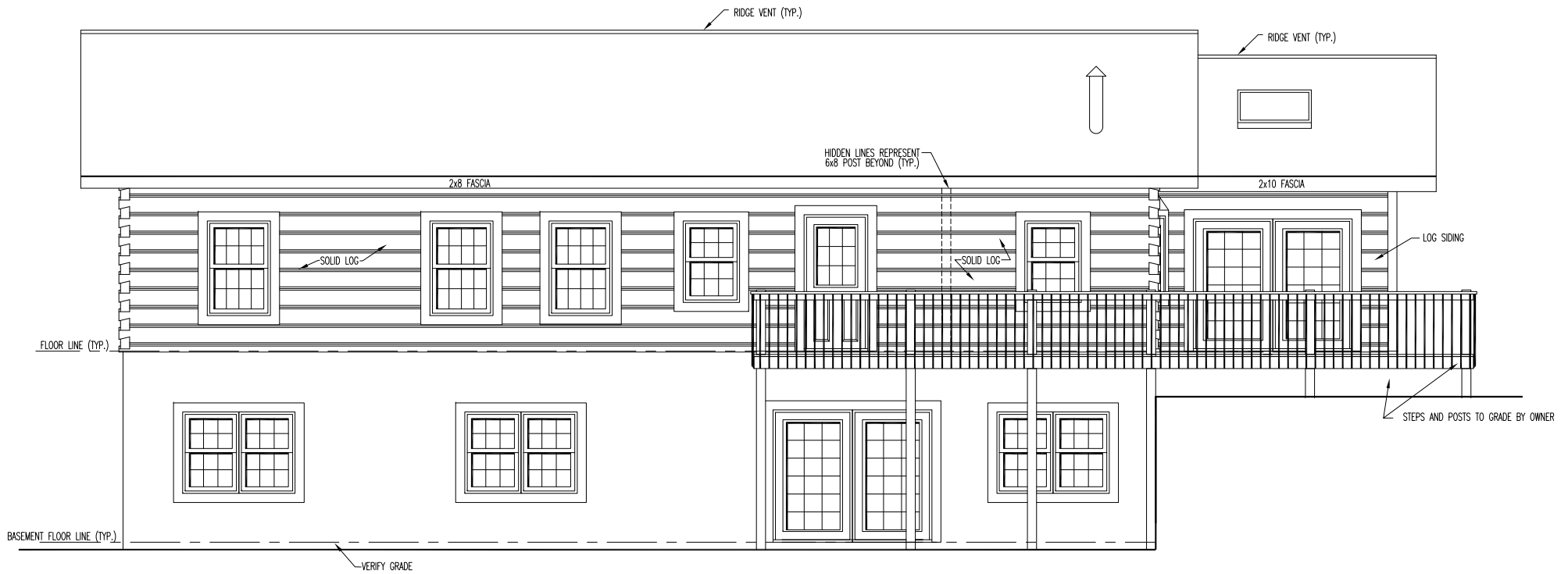
RIGHT ELEVATION
