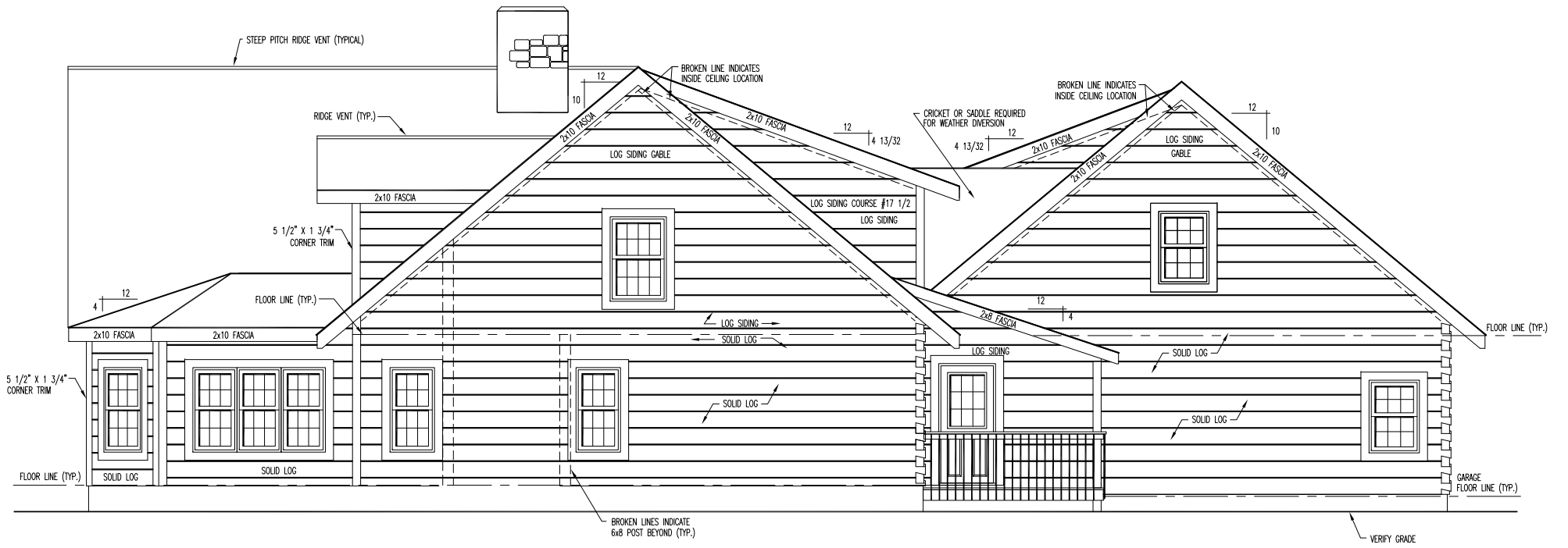
RIGHT ELEVATION
