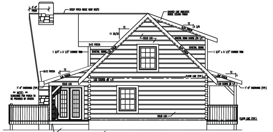
RIGHT ELEVATION
