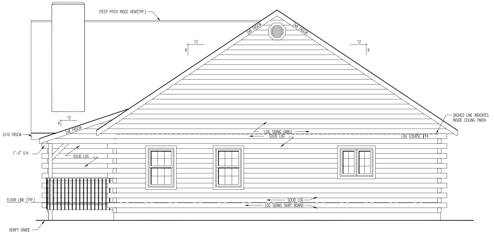
RIGHT ELEVATION
