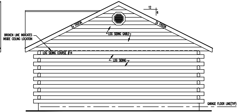
RIGHT ELEVATION
