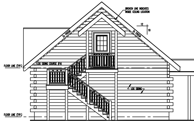
RIGHT ELEVATION
